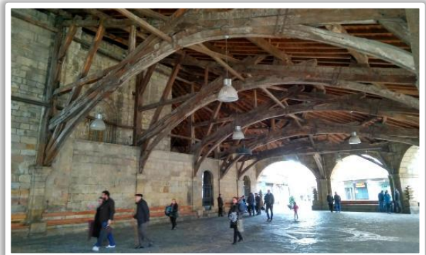
Pórtico de Santa María, construido en 1681 es el pórtico de madera con mayor luz libre conocido en Europa.
